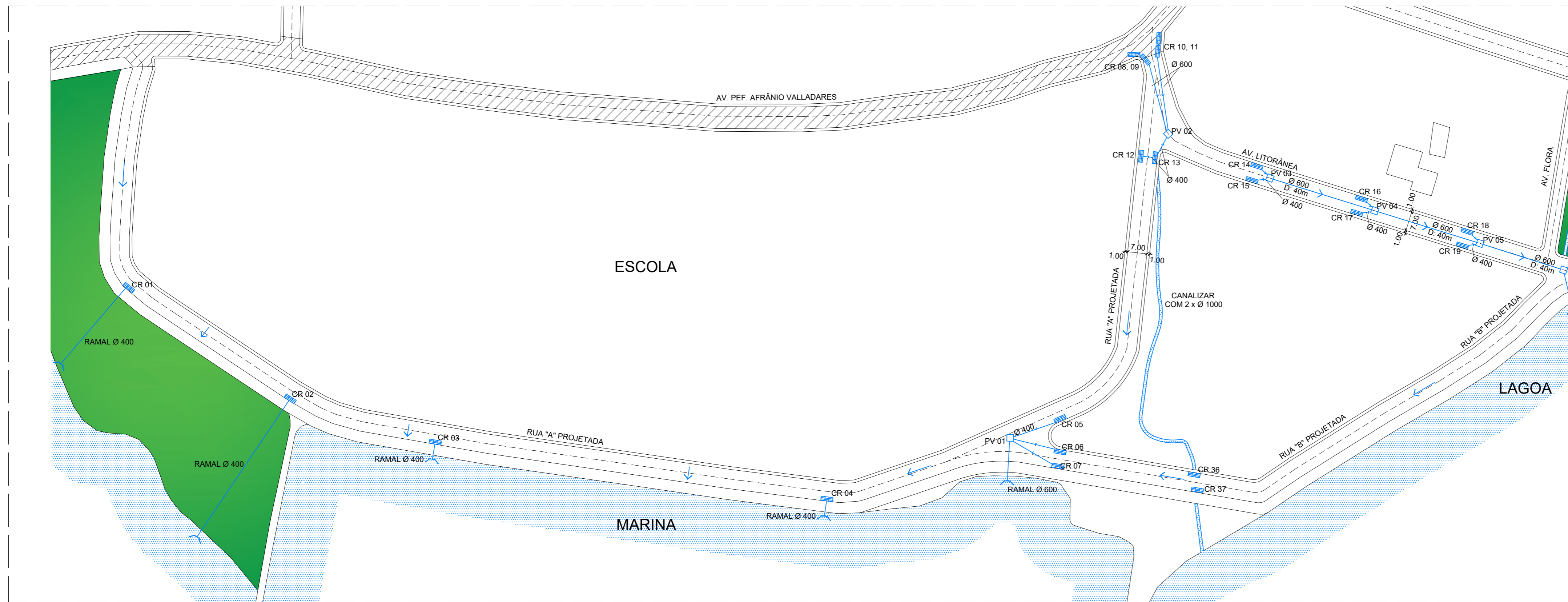
1 Planta de Drenagem - Trecho A Escala 1:1000
