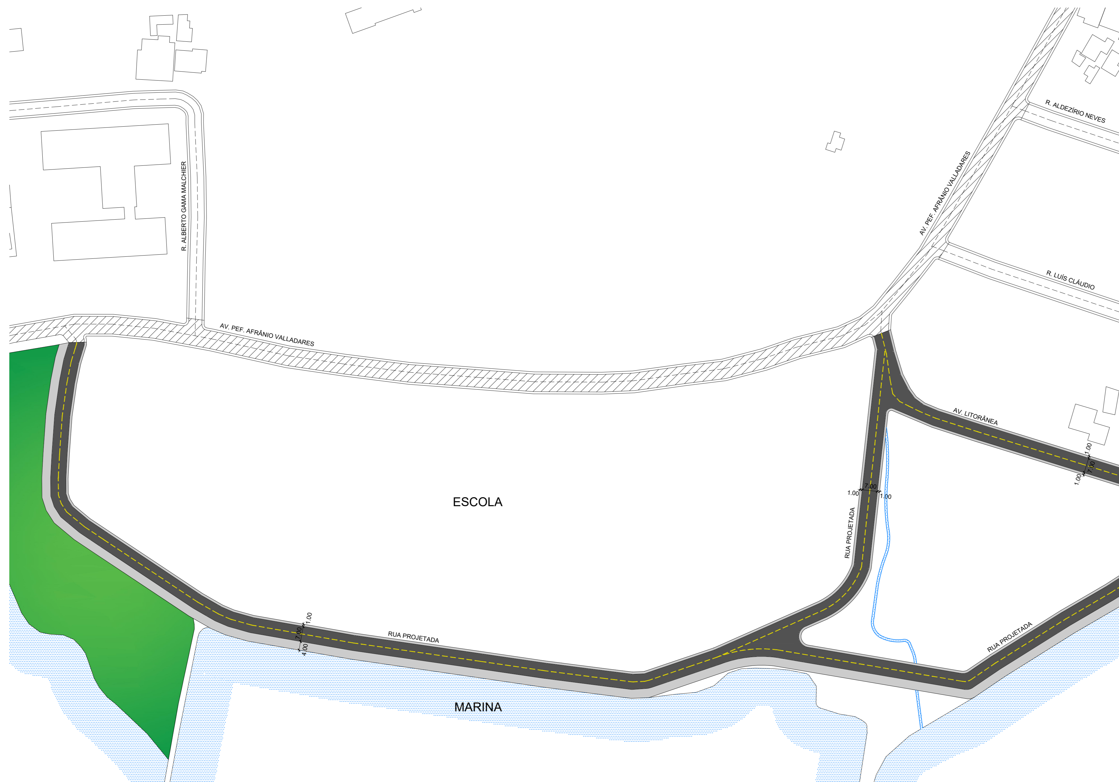
1 Planta de Pavimentação - Trecho A Escala 1:1000
