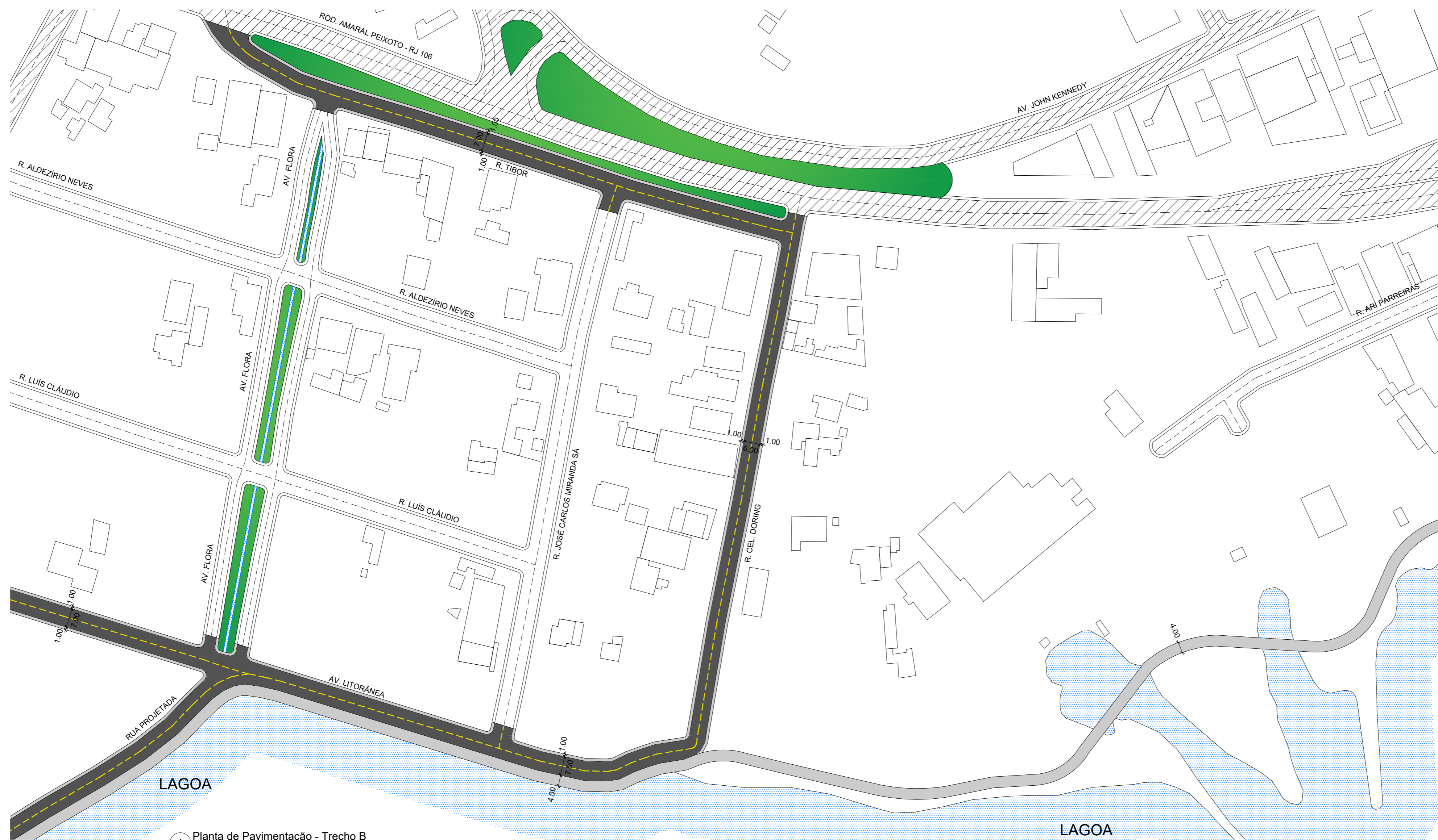
1 Planta de Pavimentação - Trecho B Escala 1:1000
