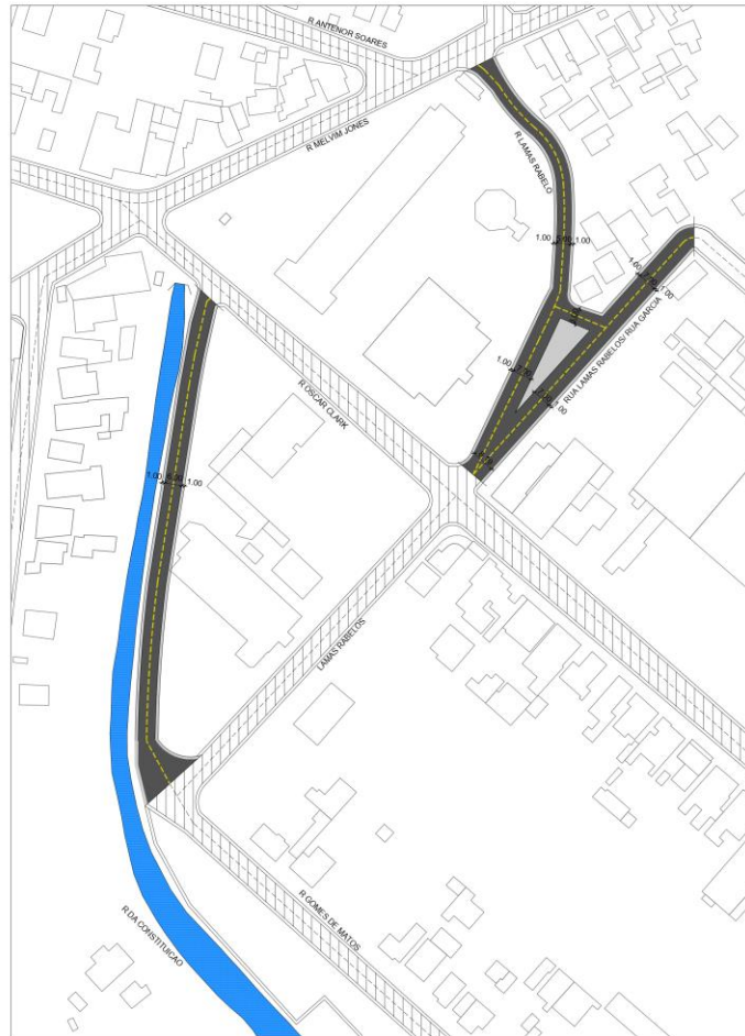
1 Planta de Pavimentação Escala 1:750
