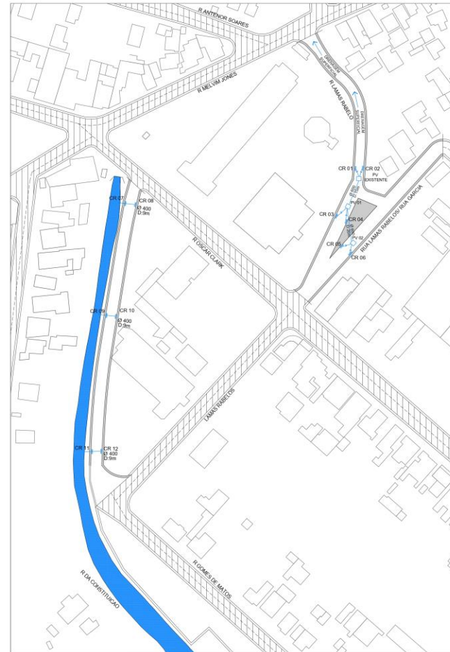
2 Planta de Drenagem Escala 1:750
